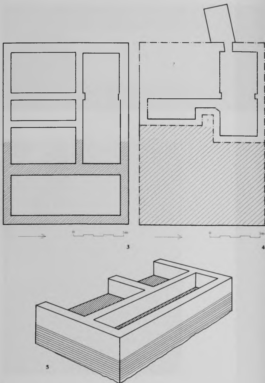
3. Villa Lante, pareti del seminterrato costituite da muratura in mattoni romani. 4. Villa Lante, cantina, la presunta estensione del muro in opus concretum . 5. Villa Lante, ricostruzione del rudere romano.
