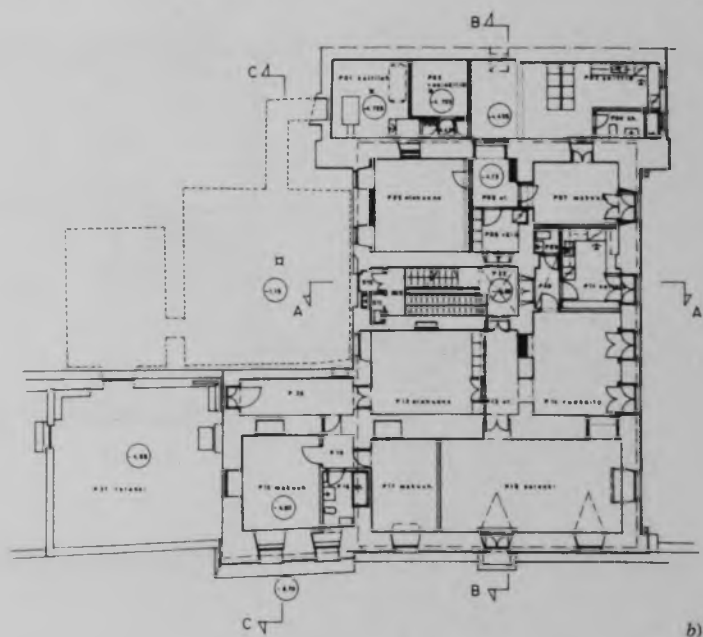
Villa Lante: a) cantina; b) seminterrato.
