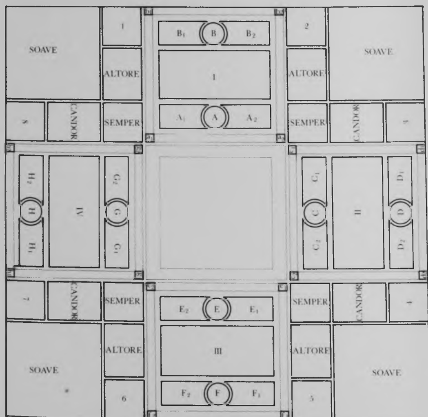
Villa Lante, piano schematico della volta del salone. - A destra il lato nord.
