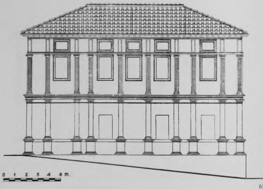
Villa Lante: a) facciata nord; b) facciata sud. Ricostruzione di A. Prandi.
