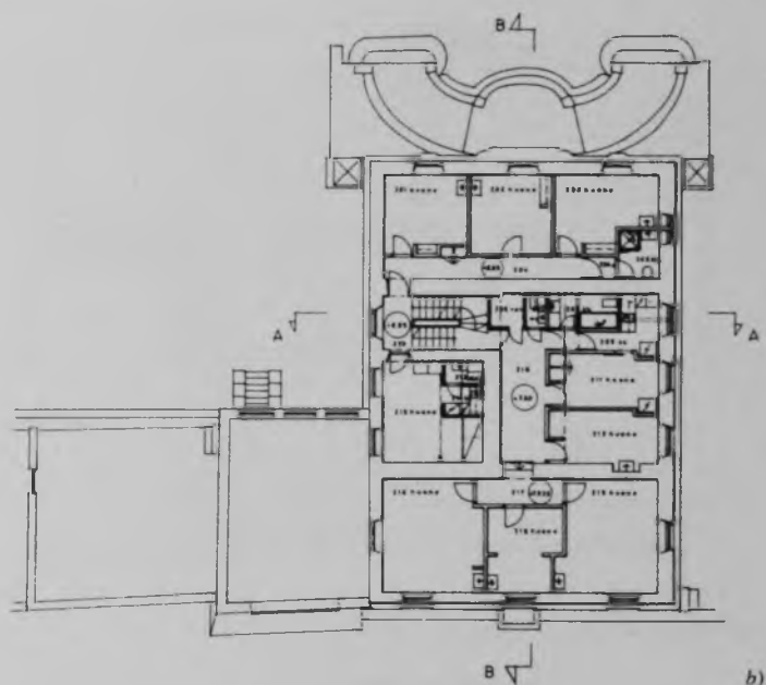
Villa Lante: a) primo piano; b) attico.
