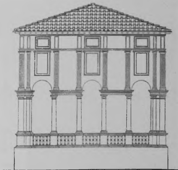
Villa Lante: a) facciata ovest; b) facciata est. Ricostruzione di A. Prandi.
