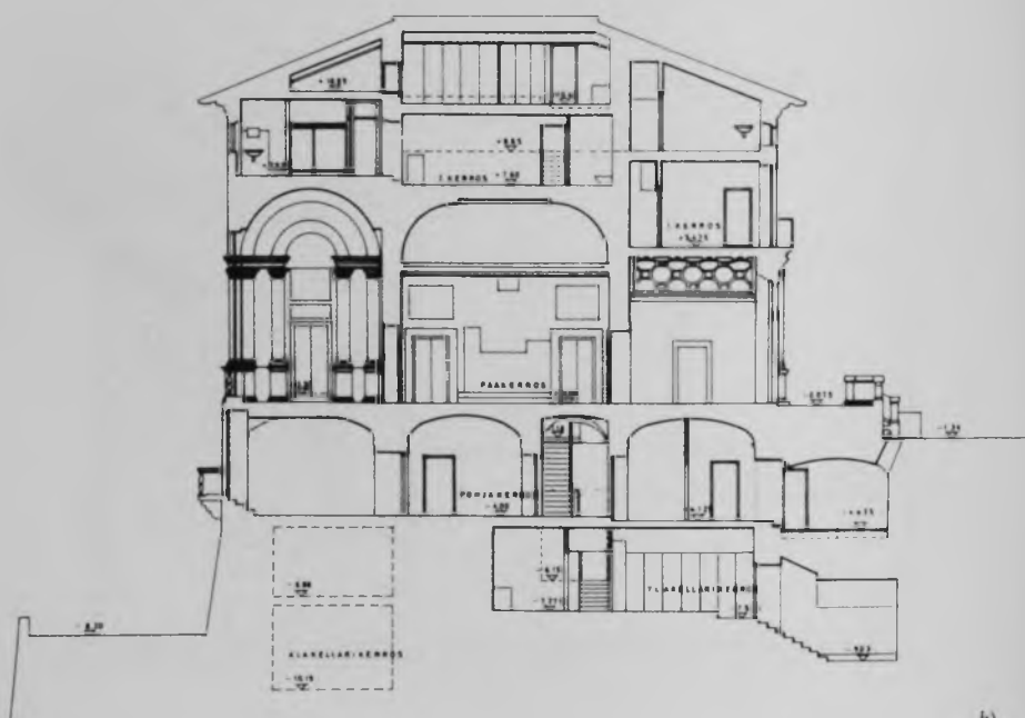
Villa Lante: a) sezione nord-sud verso est; b) sezione est-ovest verso sud.
