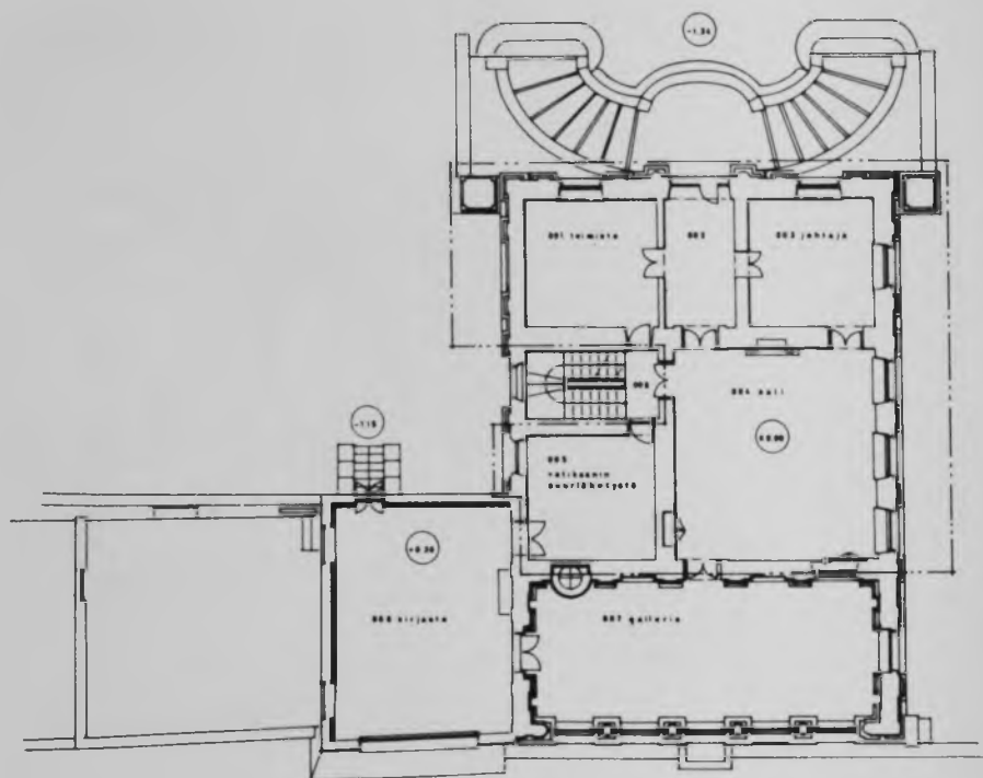
Villa Lante, piano nobile.
